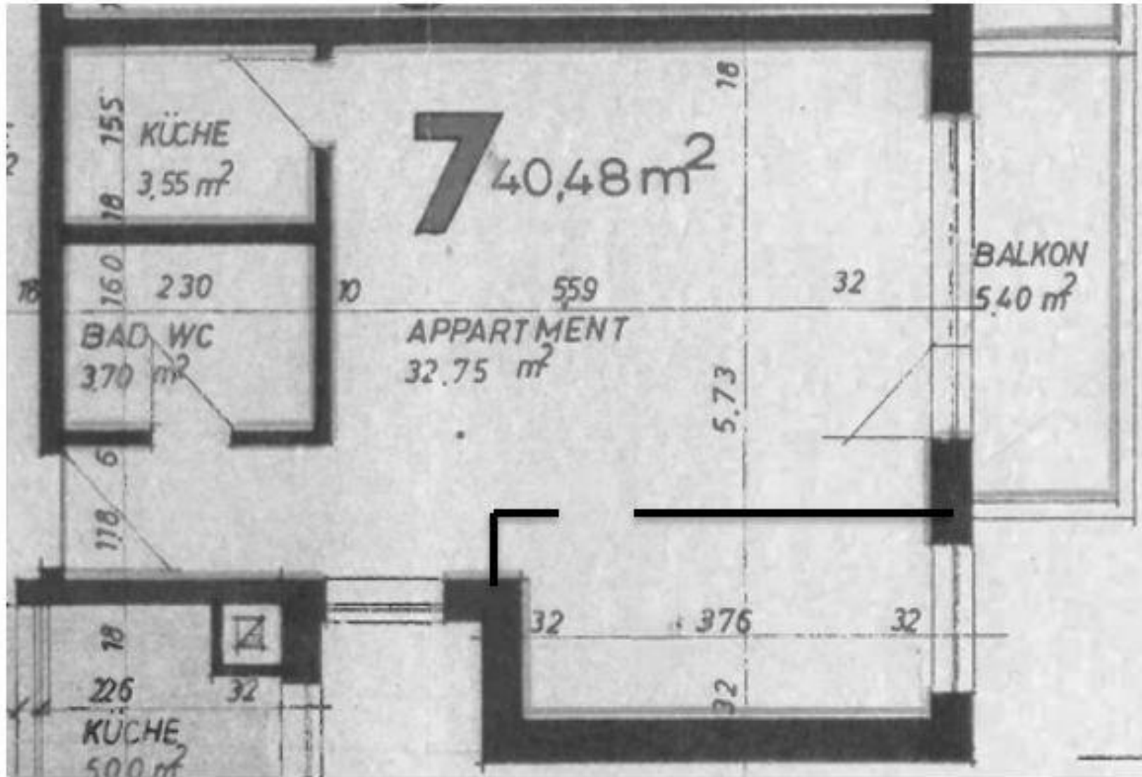
2. Obergeschoss
